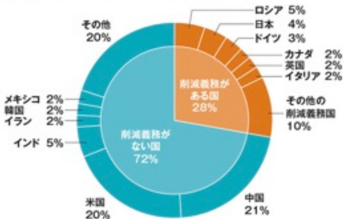
●世界のエネルギー起源CO 2 の国別排出割合(2007年)
